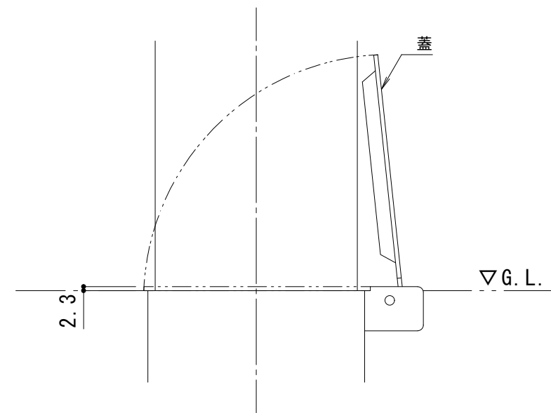
埋設管蓋部 詳細図 S = 1 : 3
