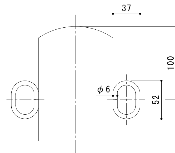
フック部詳細図 S = 1 : 3
