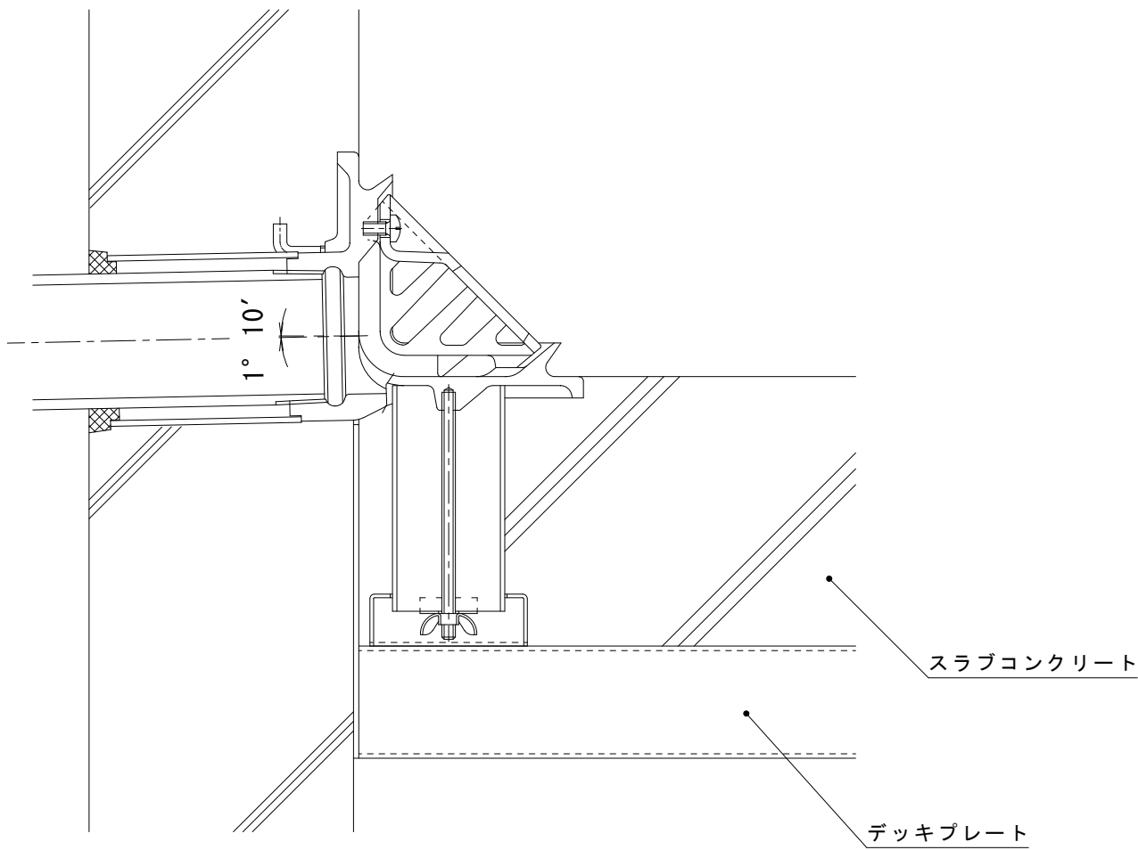
施工例 S = 1 : 3
