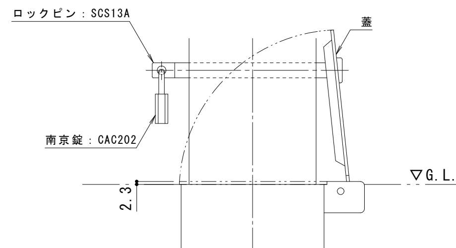
南京錠部詳細図 S = 1 : 3
