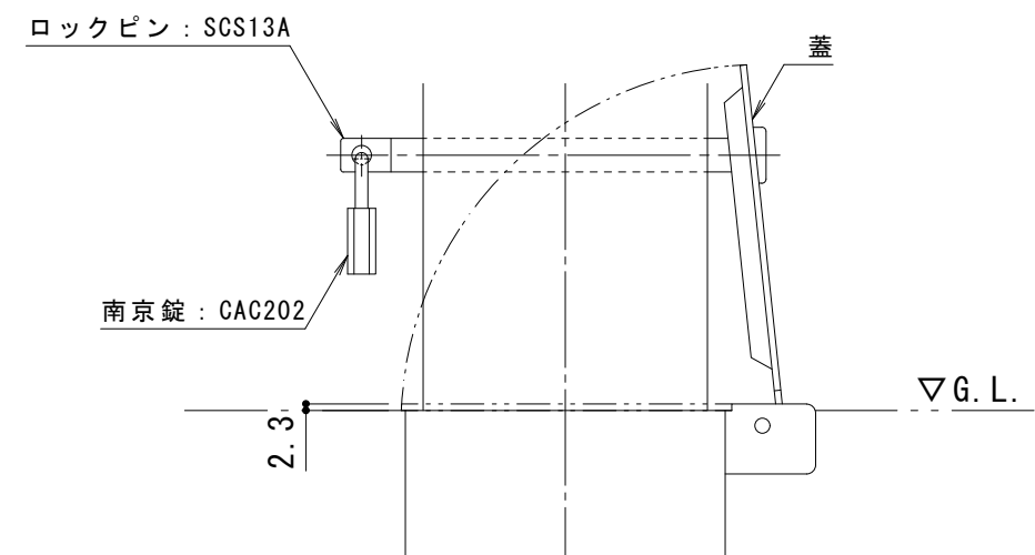
南京錠部詳細図 S = 1 : 3
