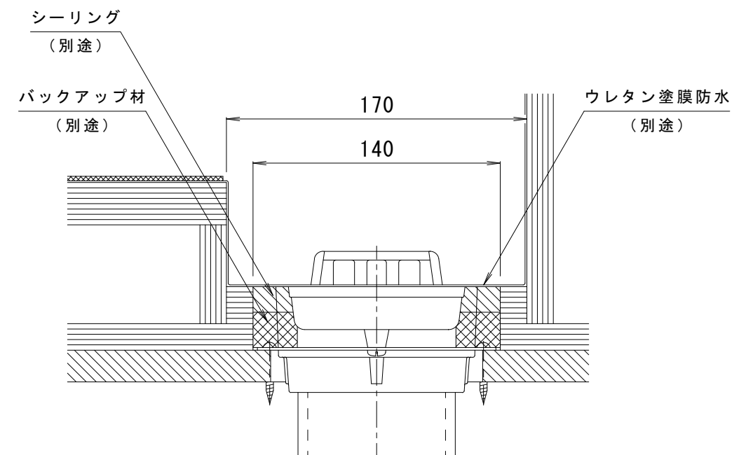
納まり図 S = 1 : 3
