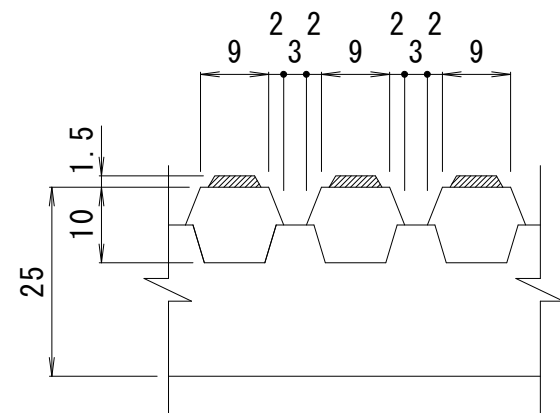
断面詳細図 1 : 1
