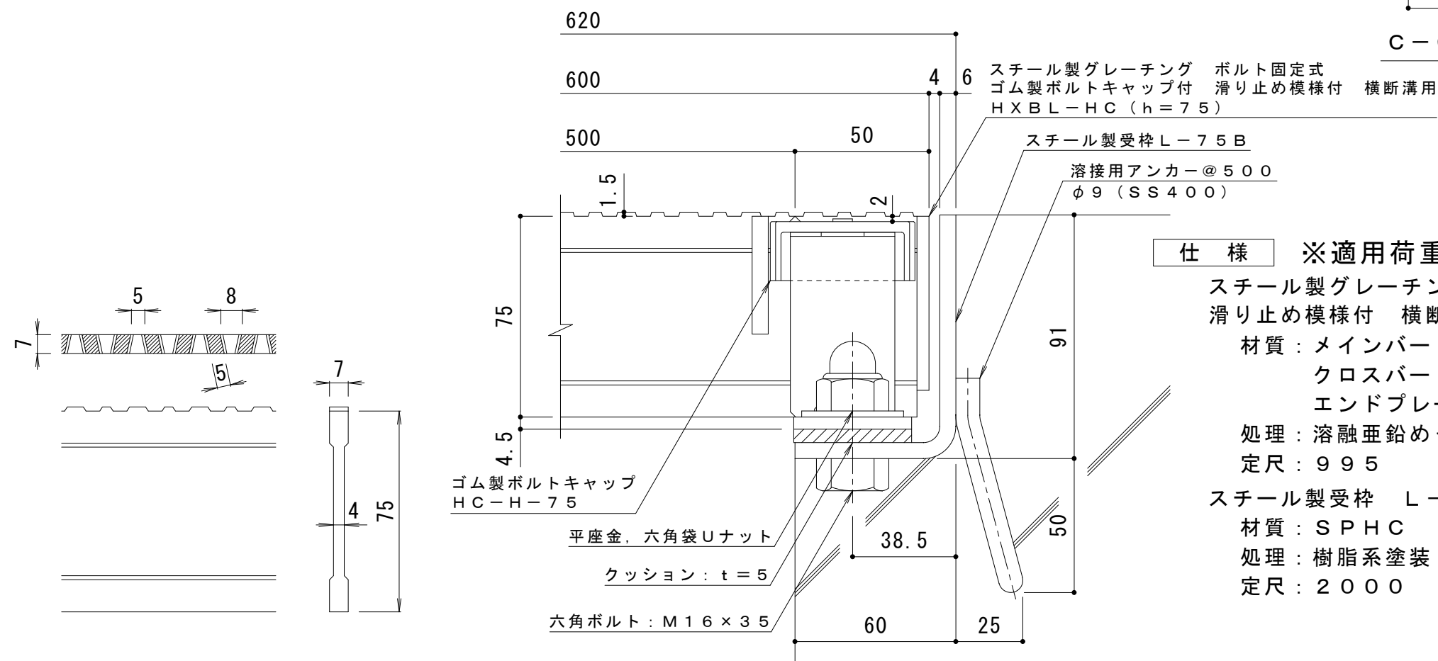
DI-75 バー形状詳細 S = 1 : 2
