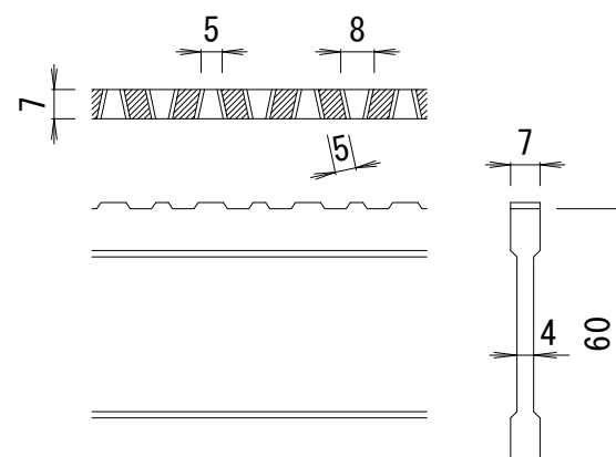
D1-60 バー形状詳細 S=1:2
