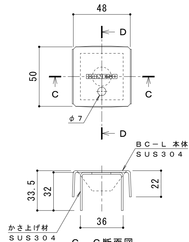
C-C断面図
