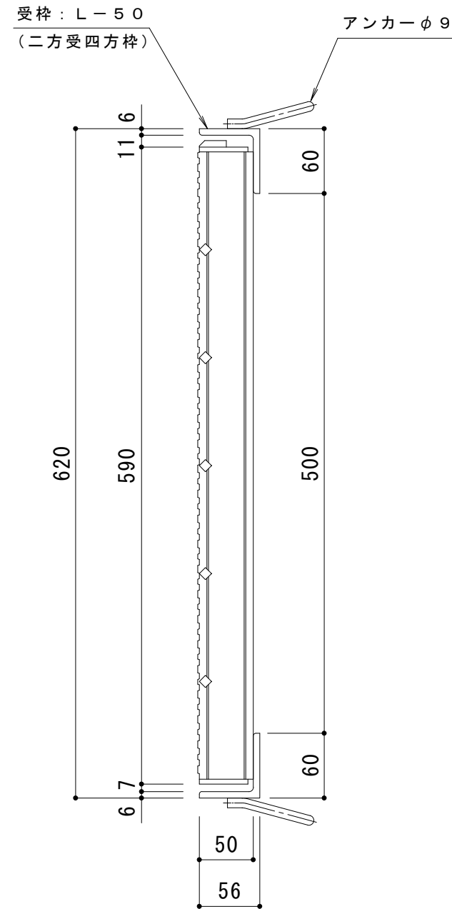
DI-50 バー形状詳細 S=1:2
