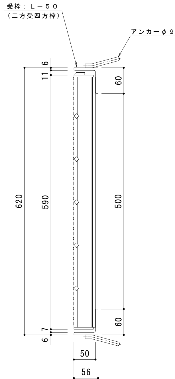
DI-50 バー形状詳細 S=1:2
