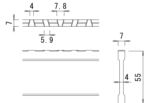
NSI-55 バー形状詳細 S=1:2
