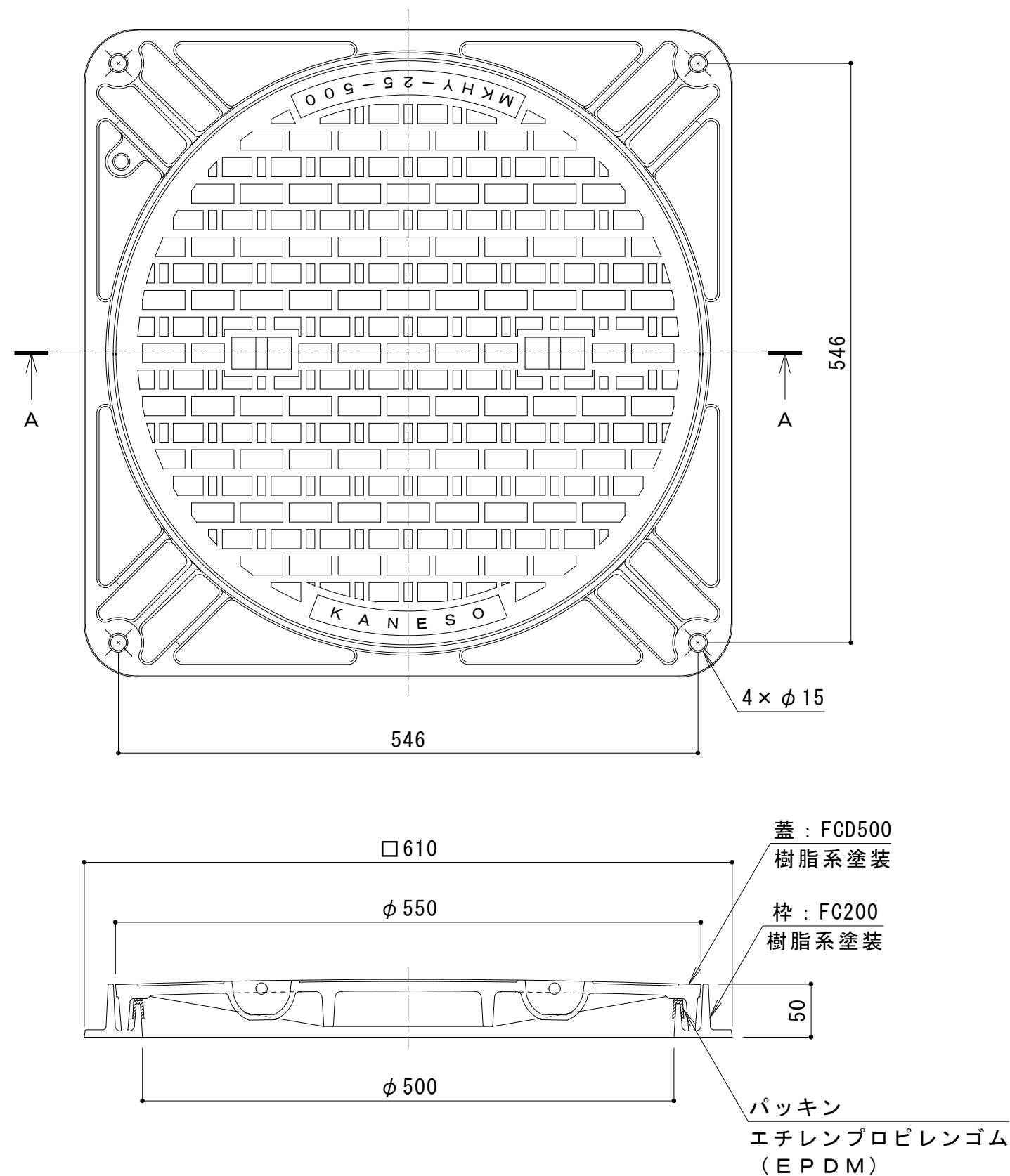
A-A断面図
