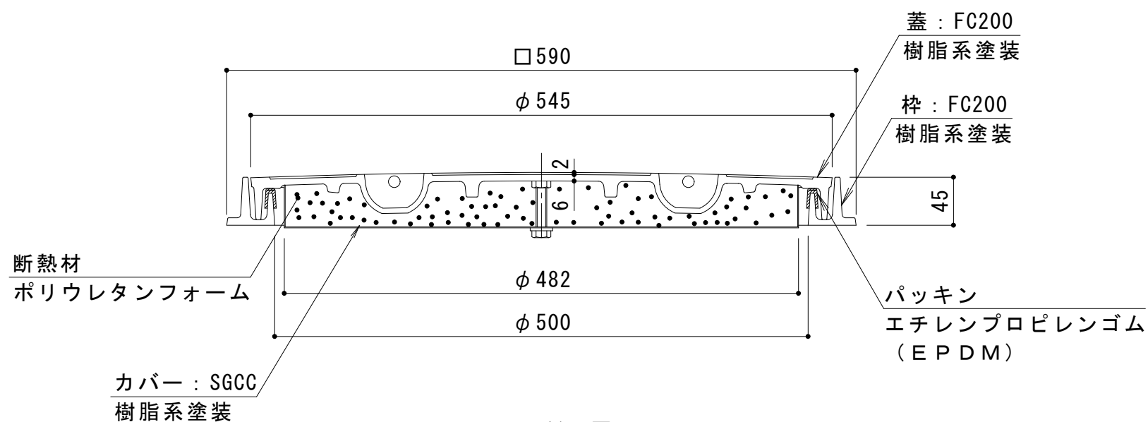
A-A断面図
