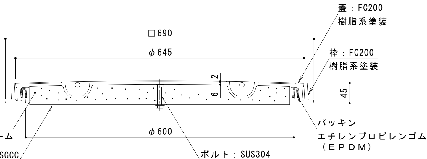
A-A断面図
