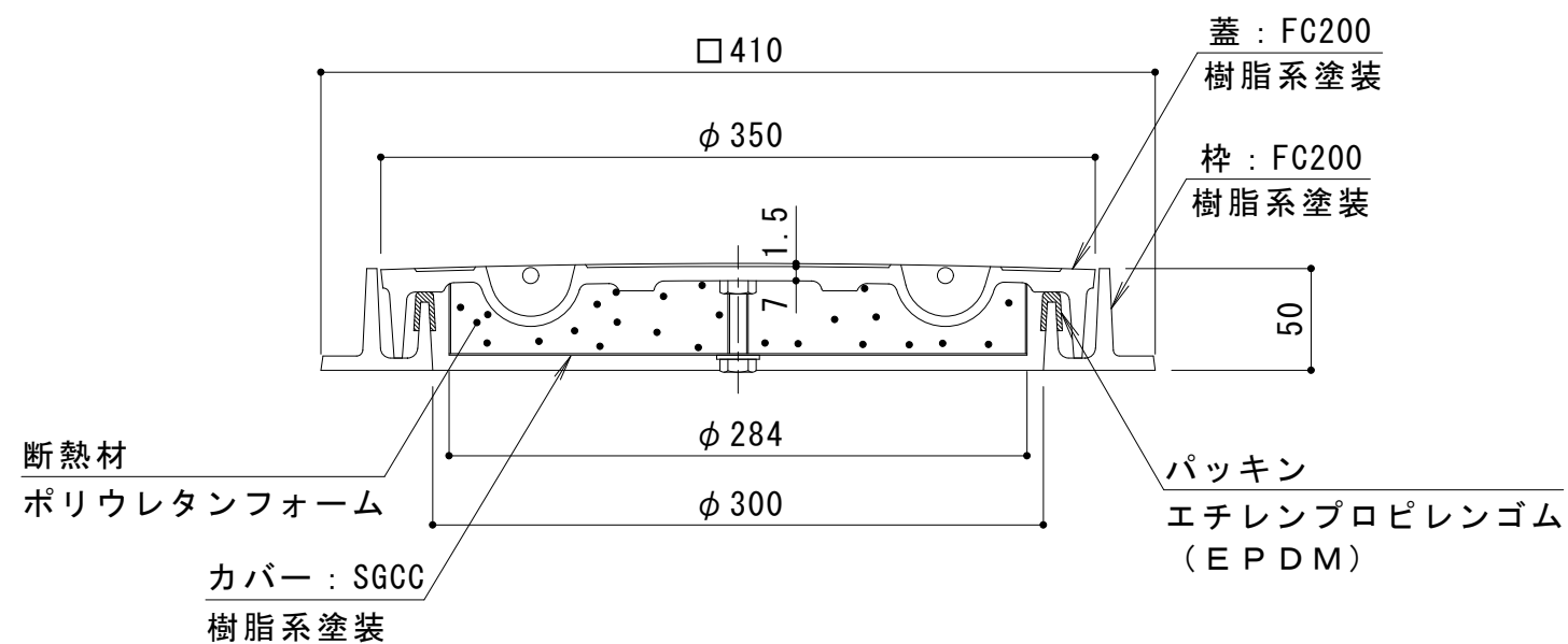
A-A断面図
