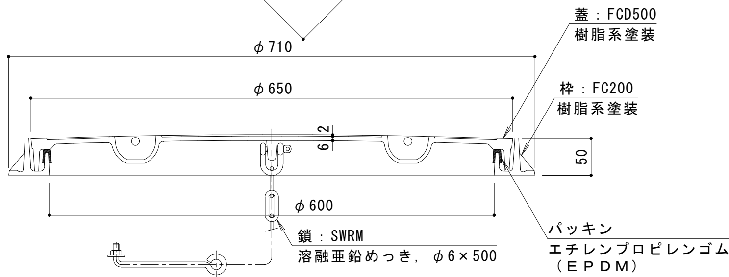
A-A断面図
