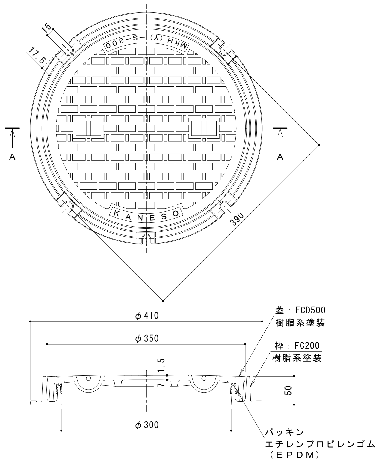
A-A断面図
