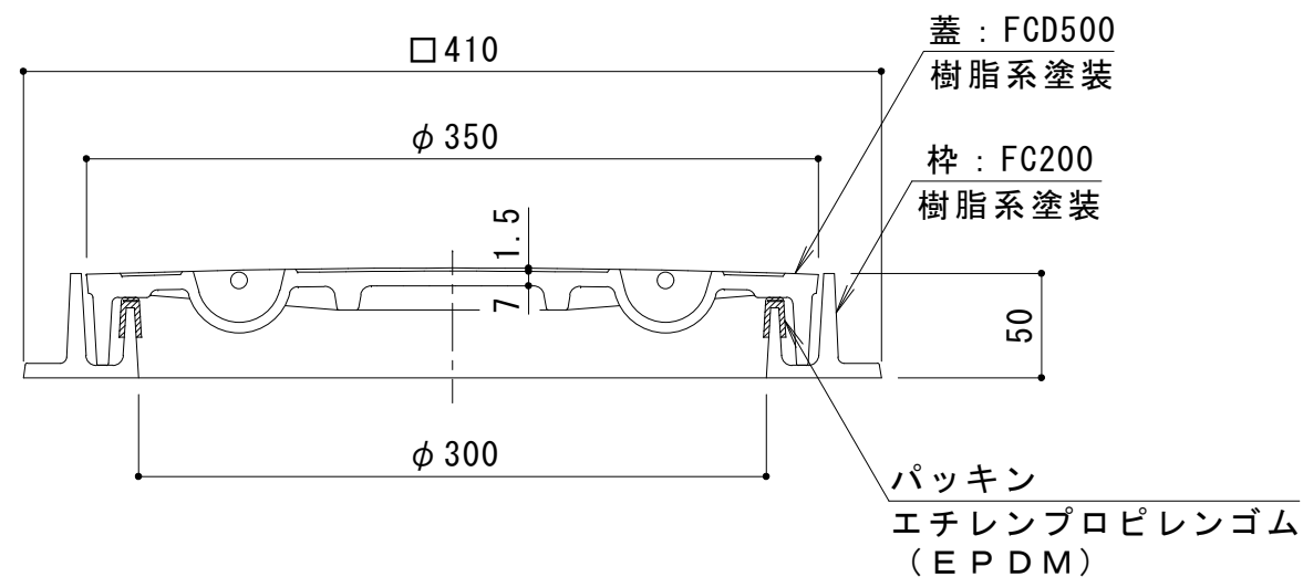
A-A断面図
