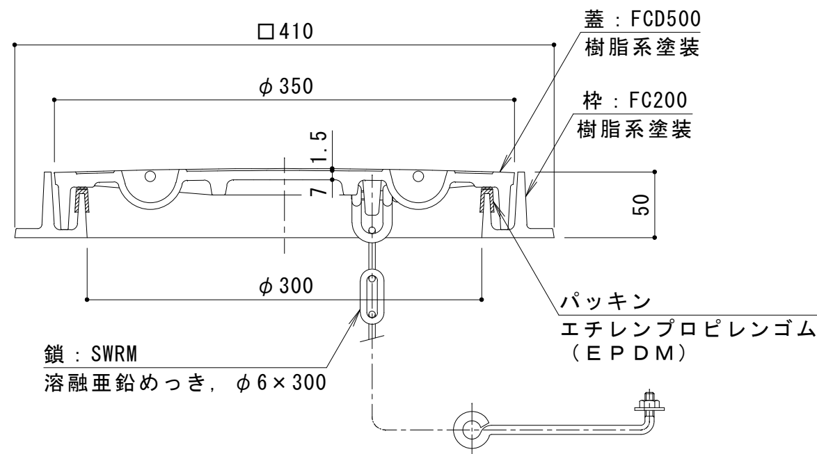
A-A断面図
