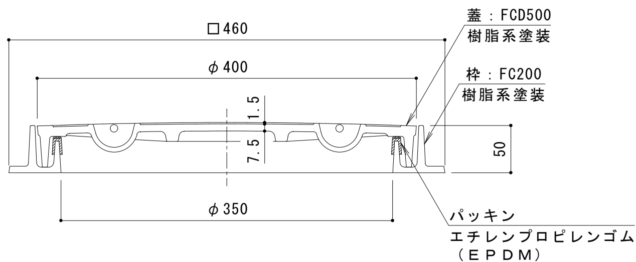
A-A断面図
