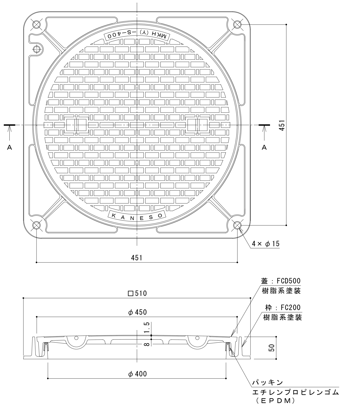
A-A断面図
