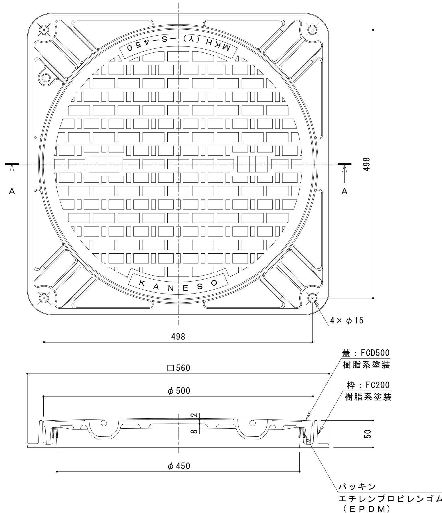
A-A 断面図
