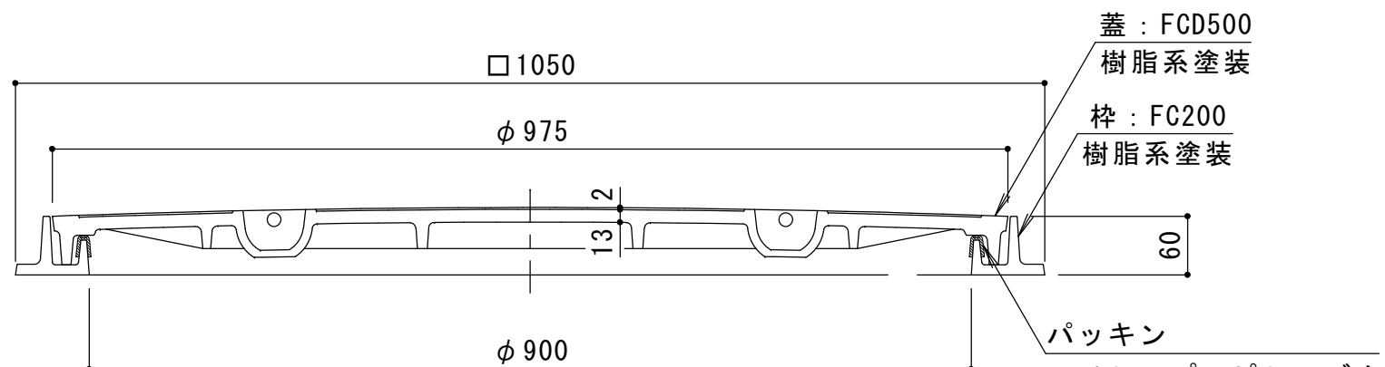
A-A断面図
