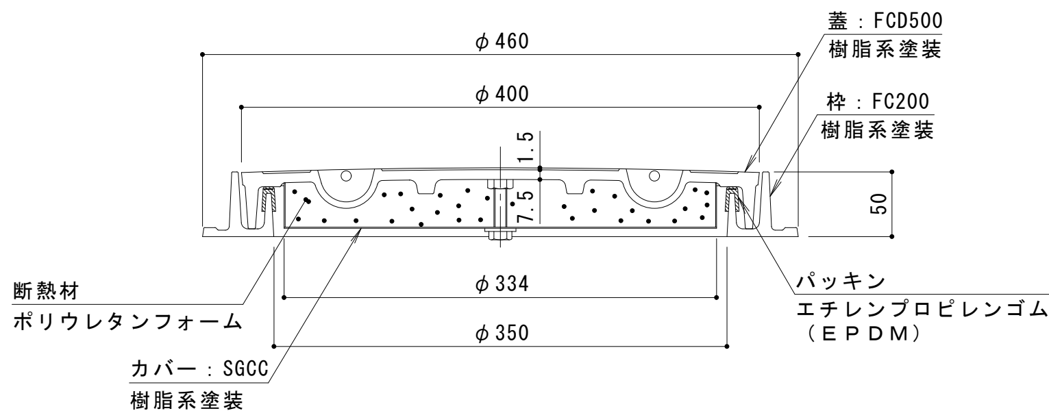
A-A断面図
