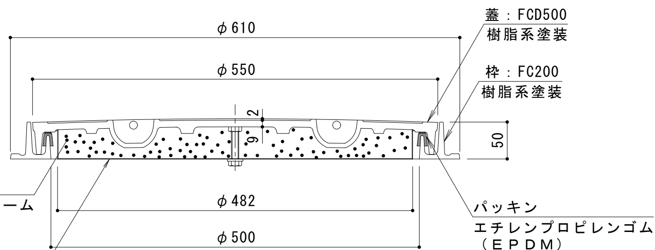
A-A断面図
