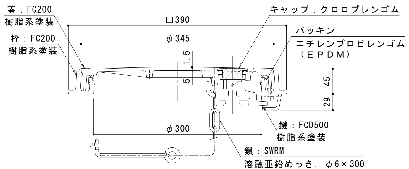
A-A断面図
