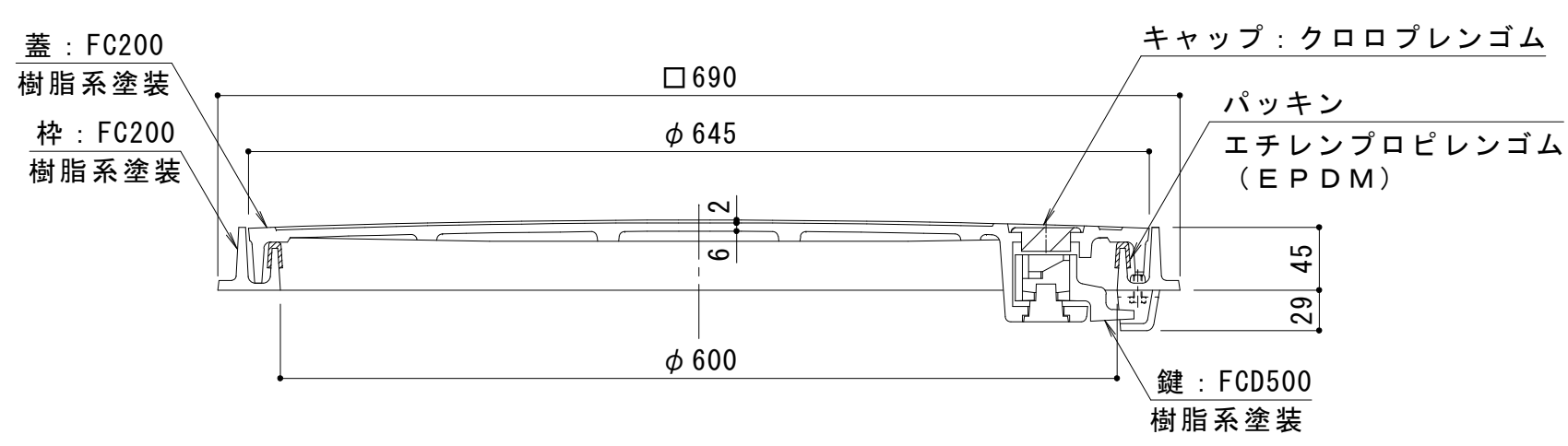
A-A 断面図
