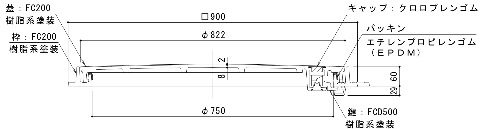
A-A断面図
