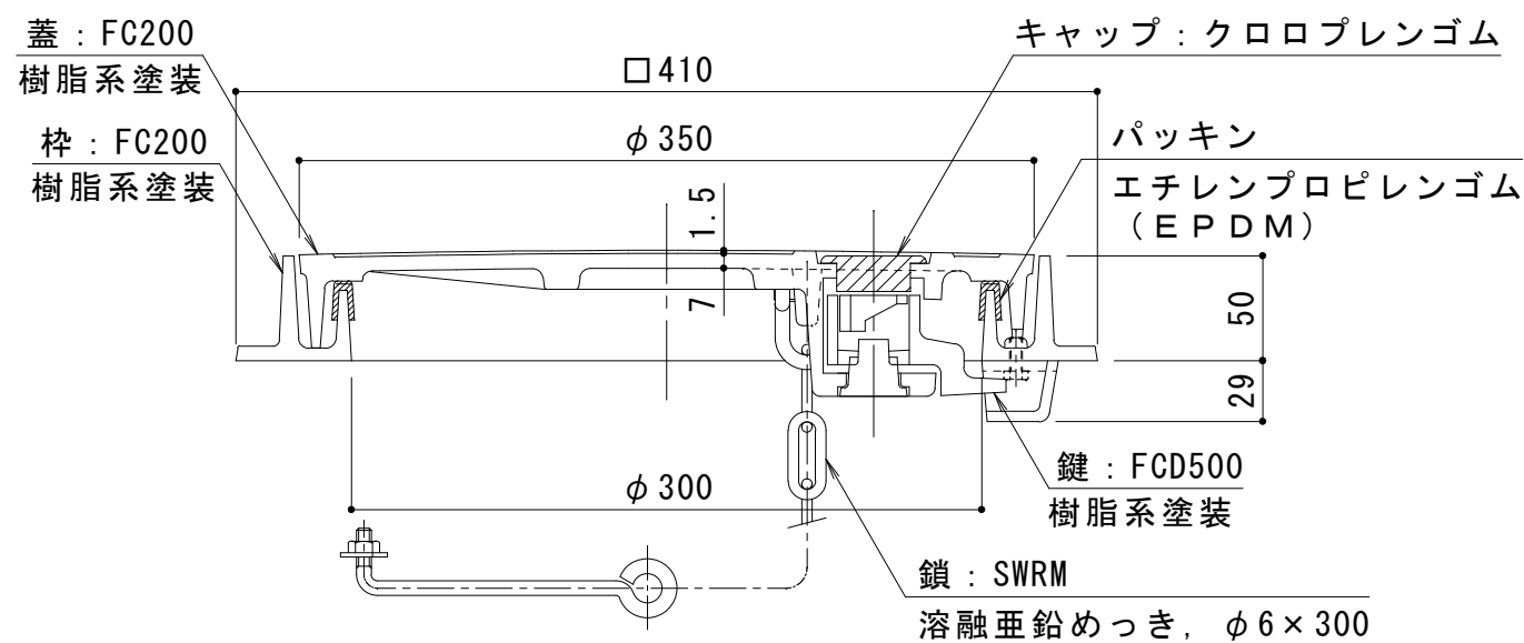
A-A断面図
