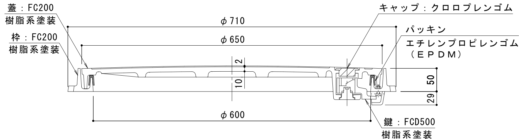
A-A断面図
