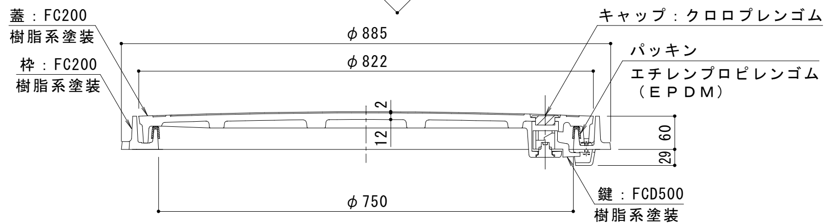
A-A断面図
