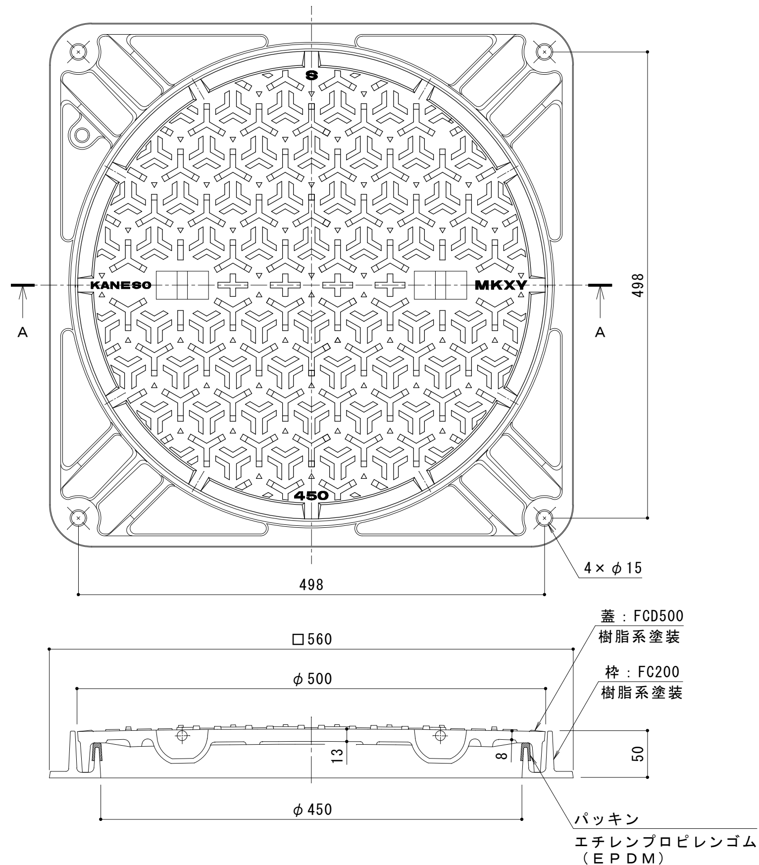
A-A断面図
