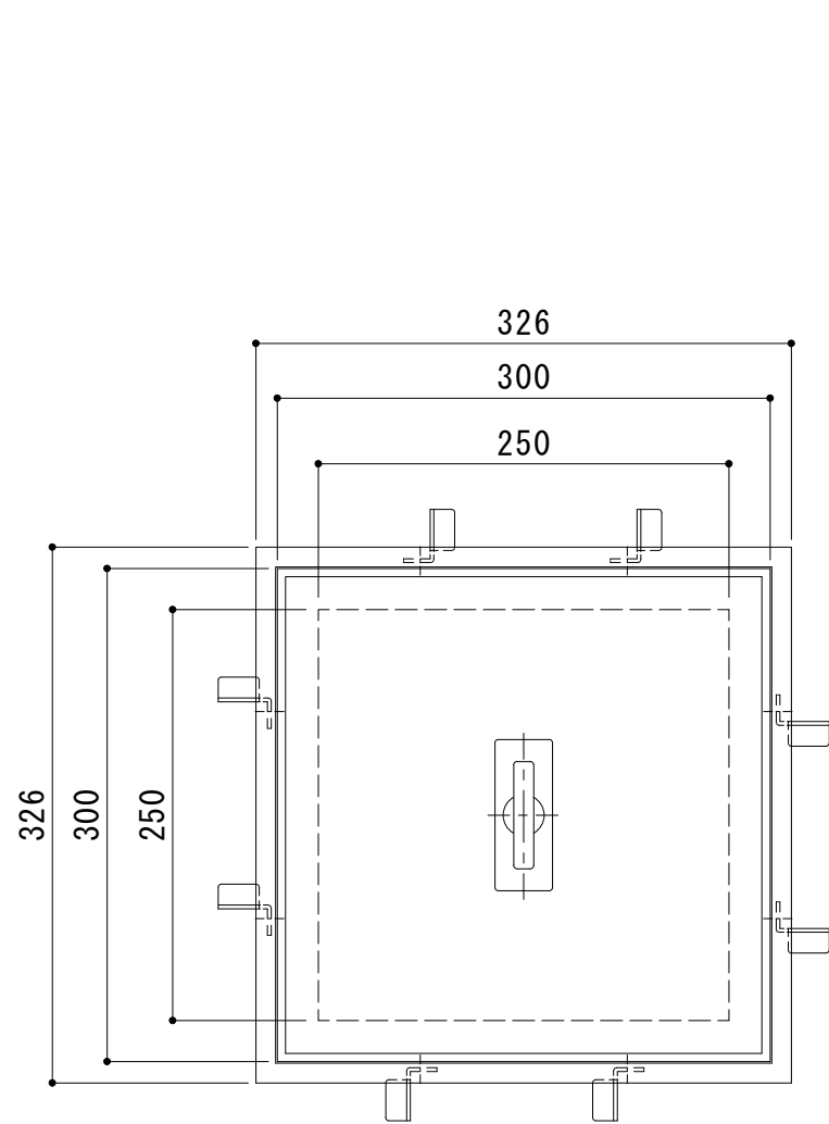
平面詳細図 S = 1 : 5
