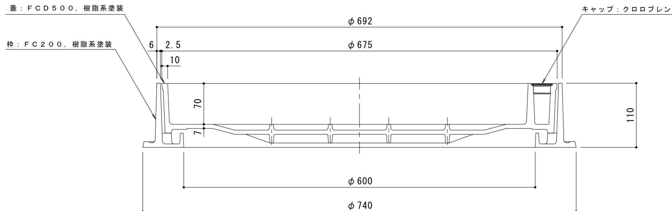
A-A 断面図 S=1:4
