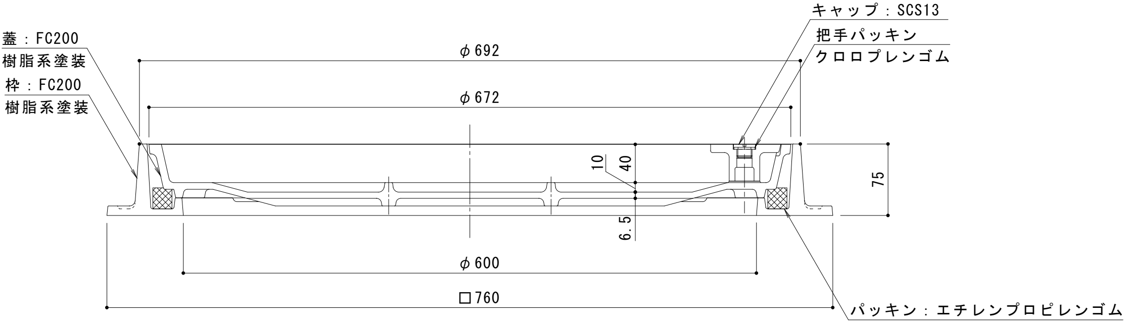
A-A断面図 S=1:4
