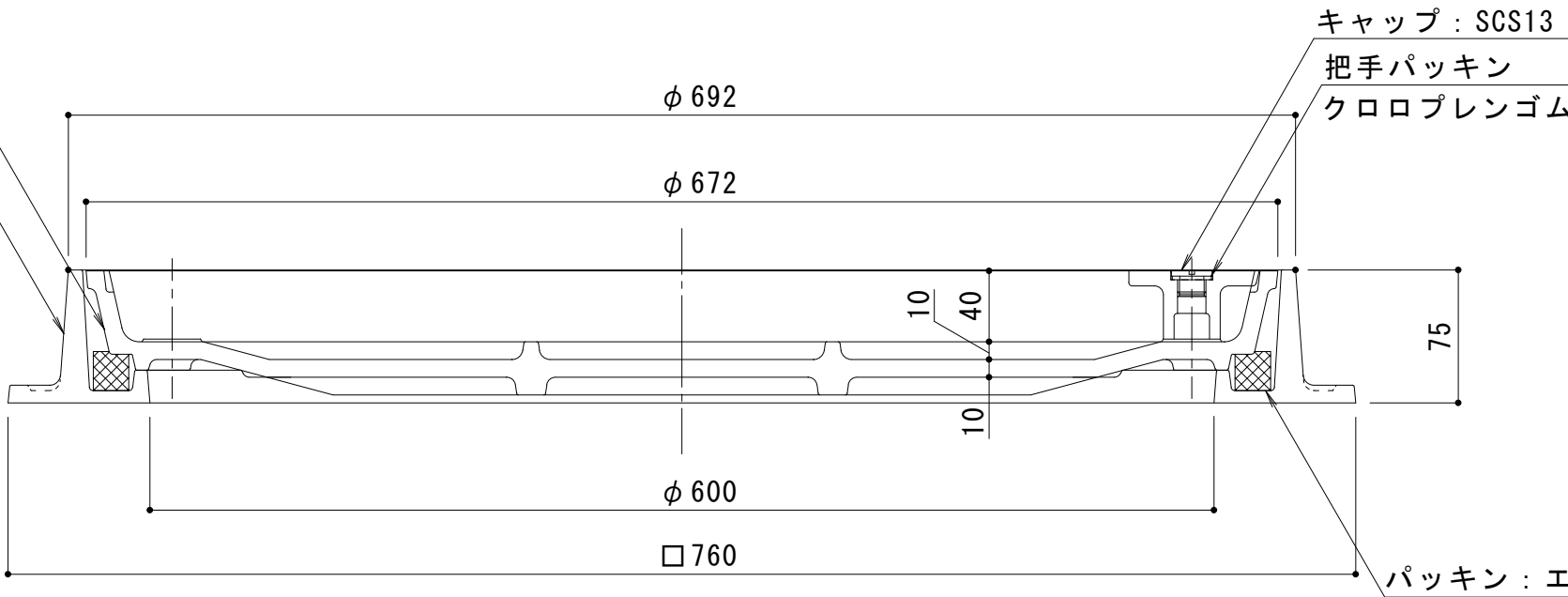
A－A断面図 S＝1：4
