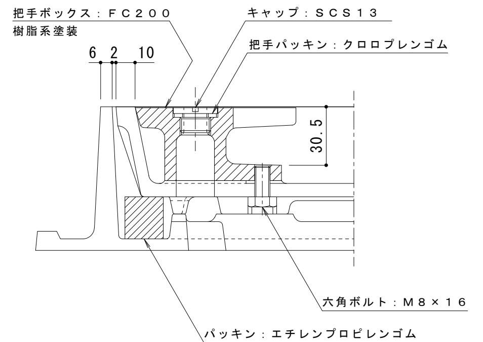
B－B'断面図 S = 1 : 2
