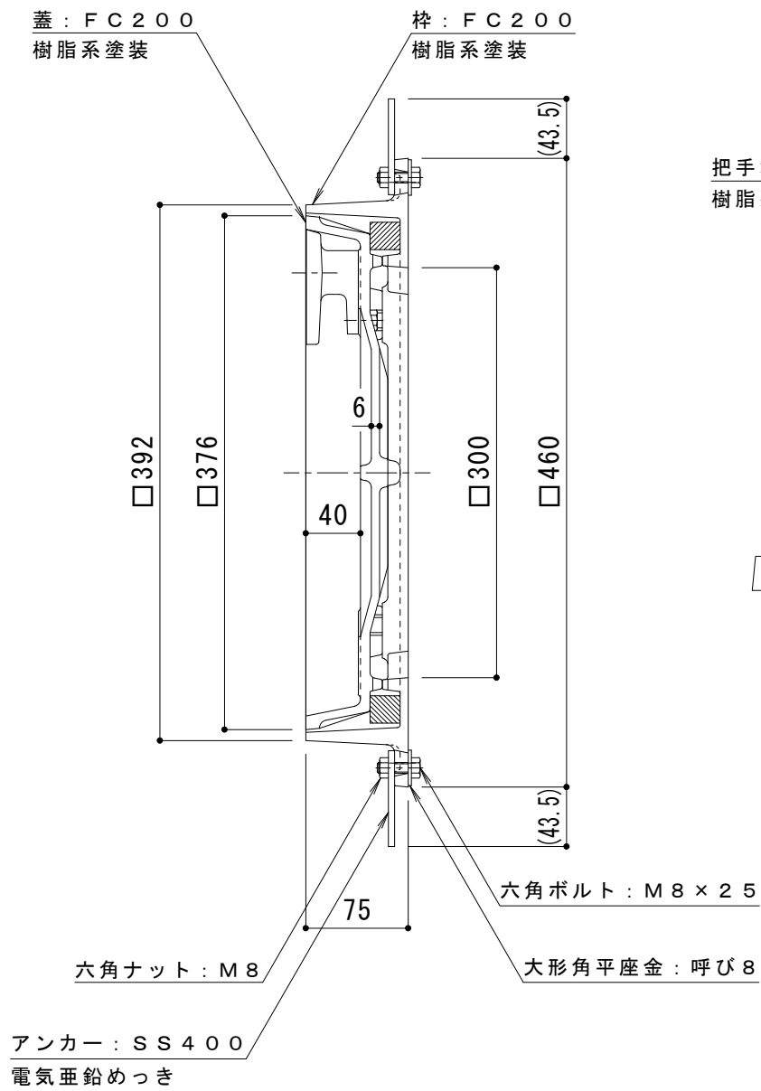
A－A'断面図 S = 1 : 5
