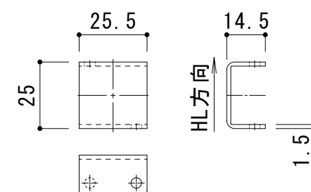
キャップ詳細図
