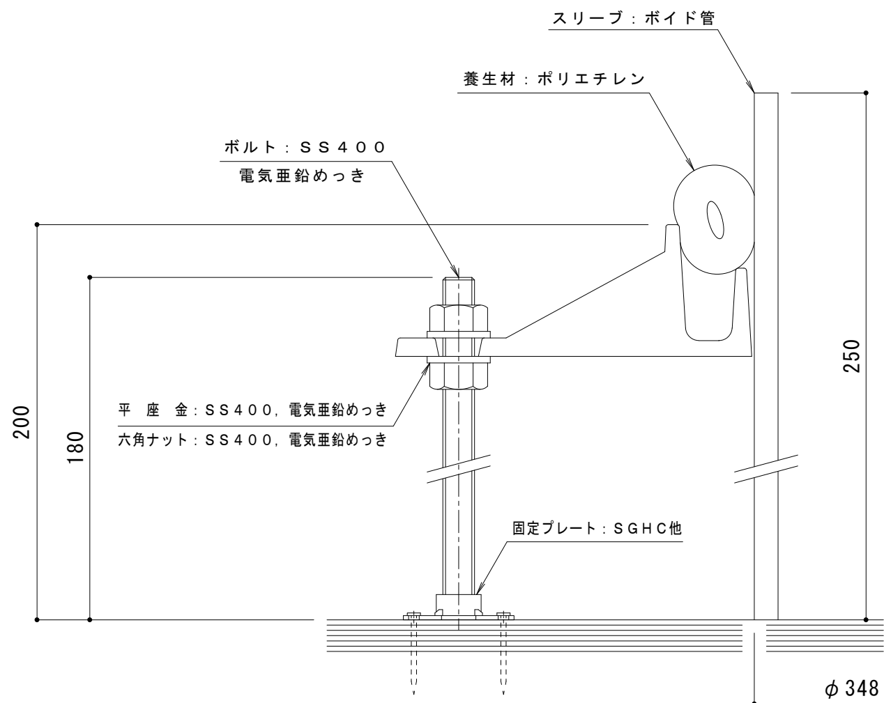
A-A' 断面図 S = 1 : 2
