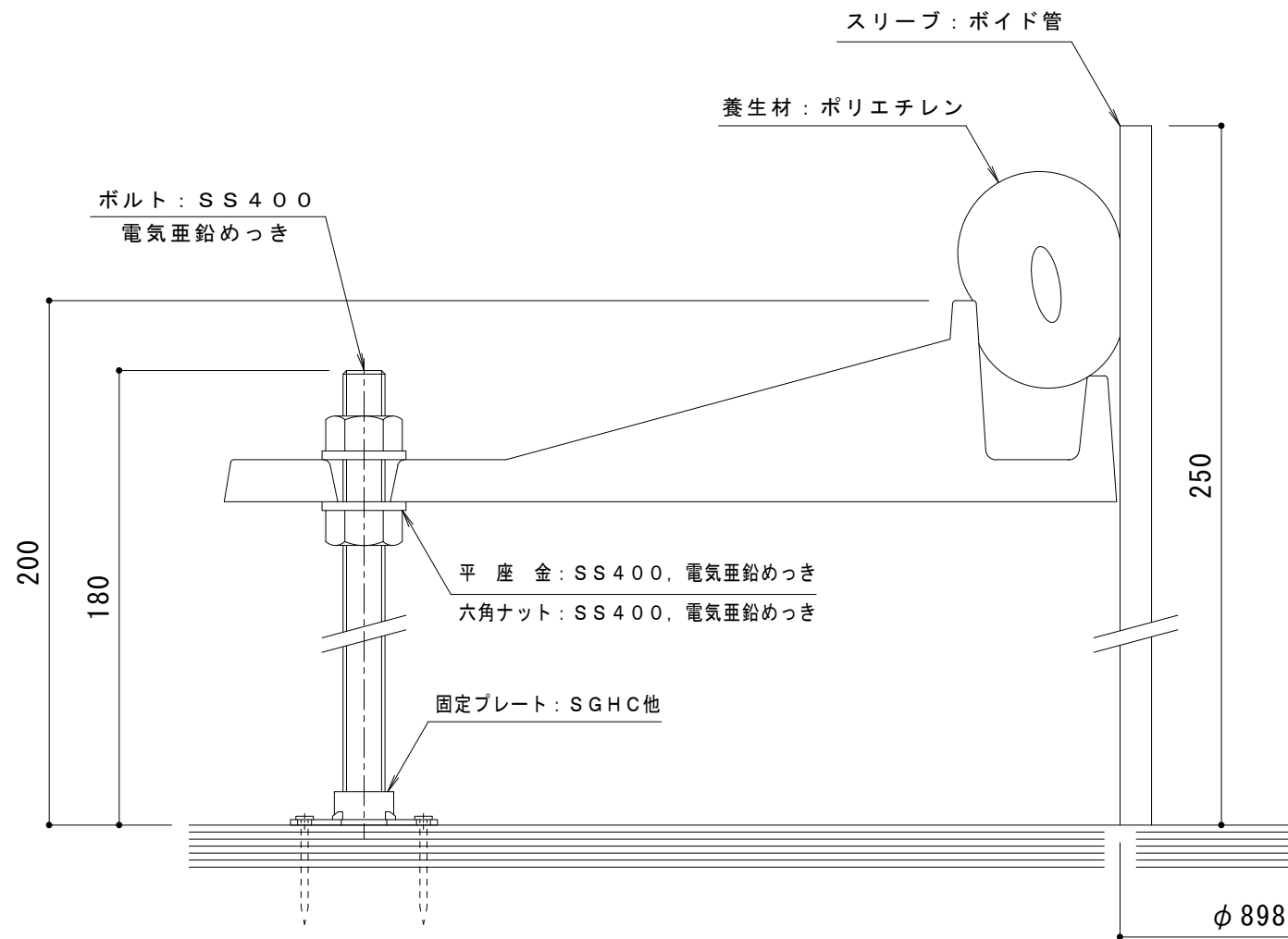
A-A' 断面図 S=1:2
