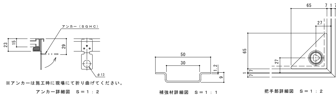
アンカー詳細図 S = 1 : 2
