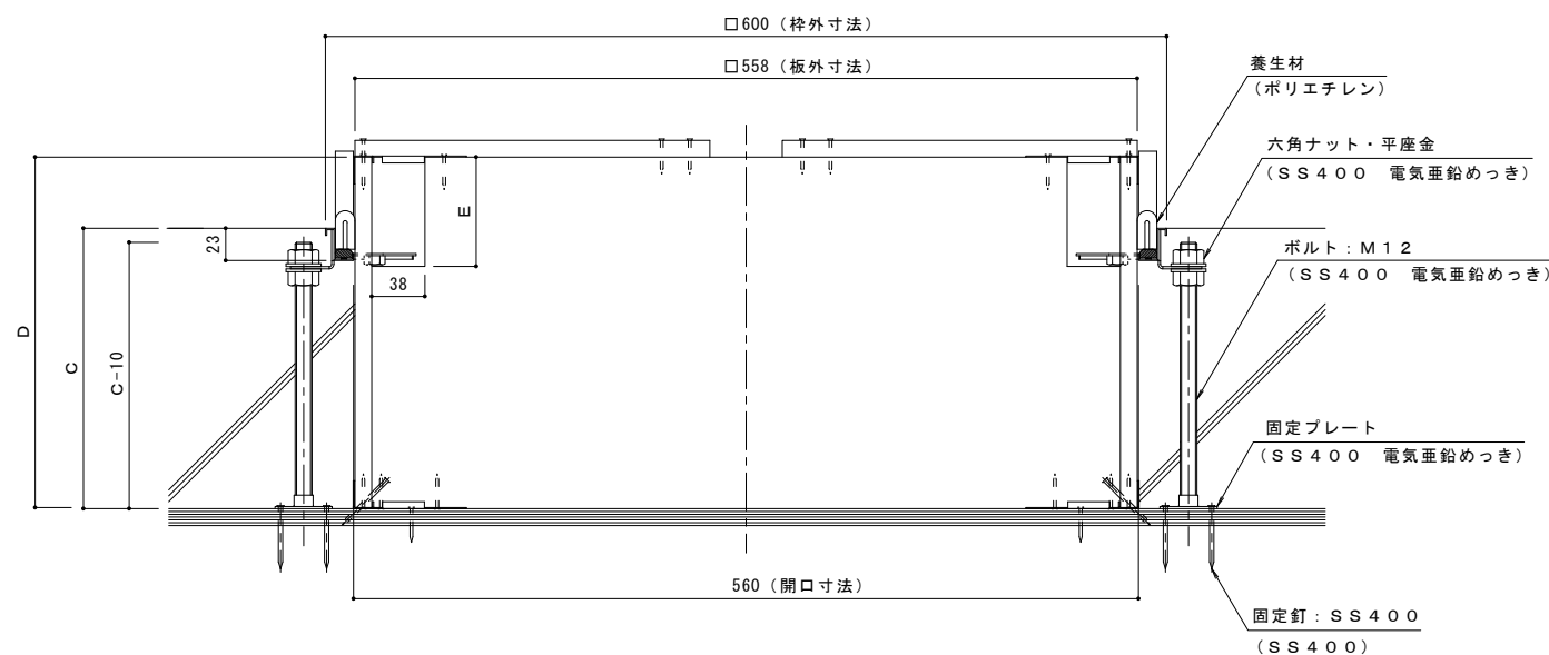
打込金具 納まり図 S = 1 : 3
