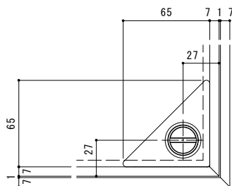
把手部詳細図 S = 1 : 2
