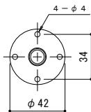
固定プレート平面図 S = 1 : 2
