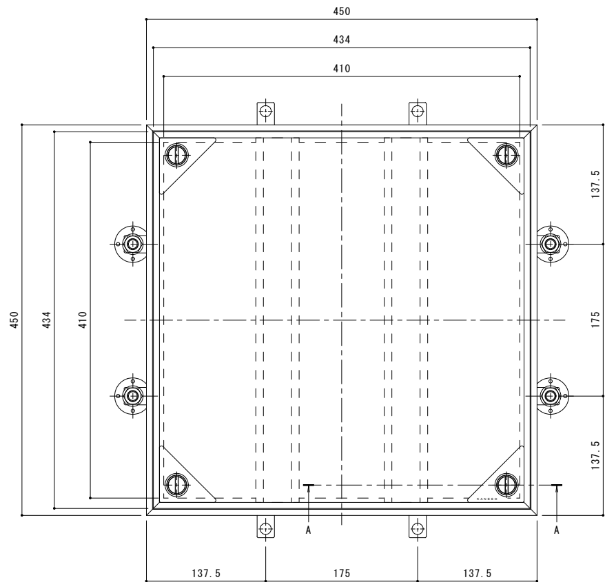
平面図 S = 1 : 3
