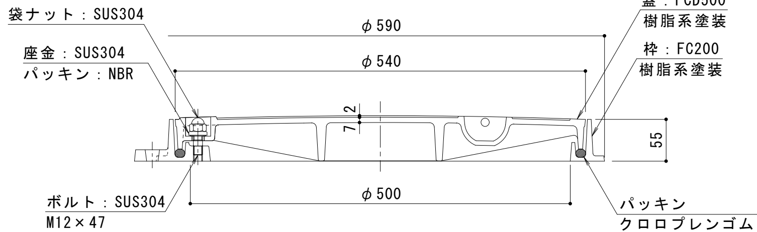
A-A 断面図
