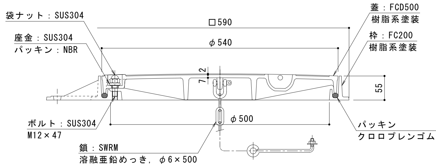
A-A 断面図
