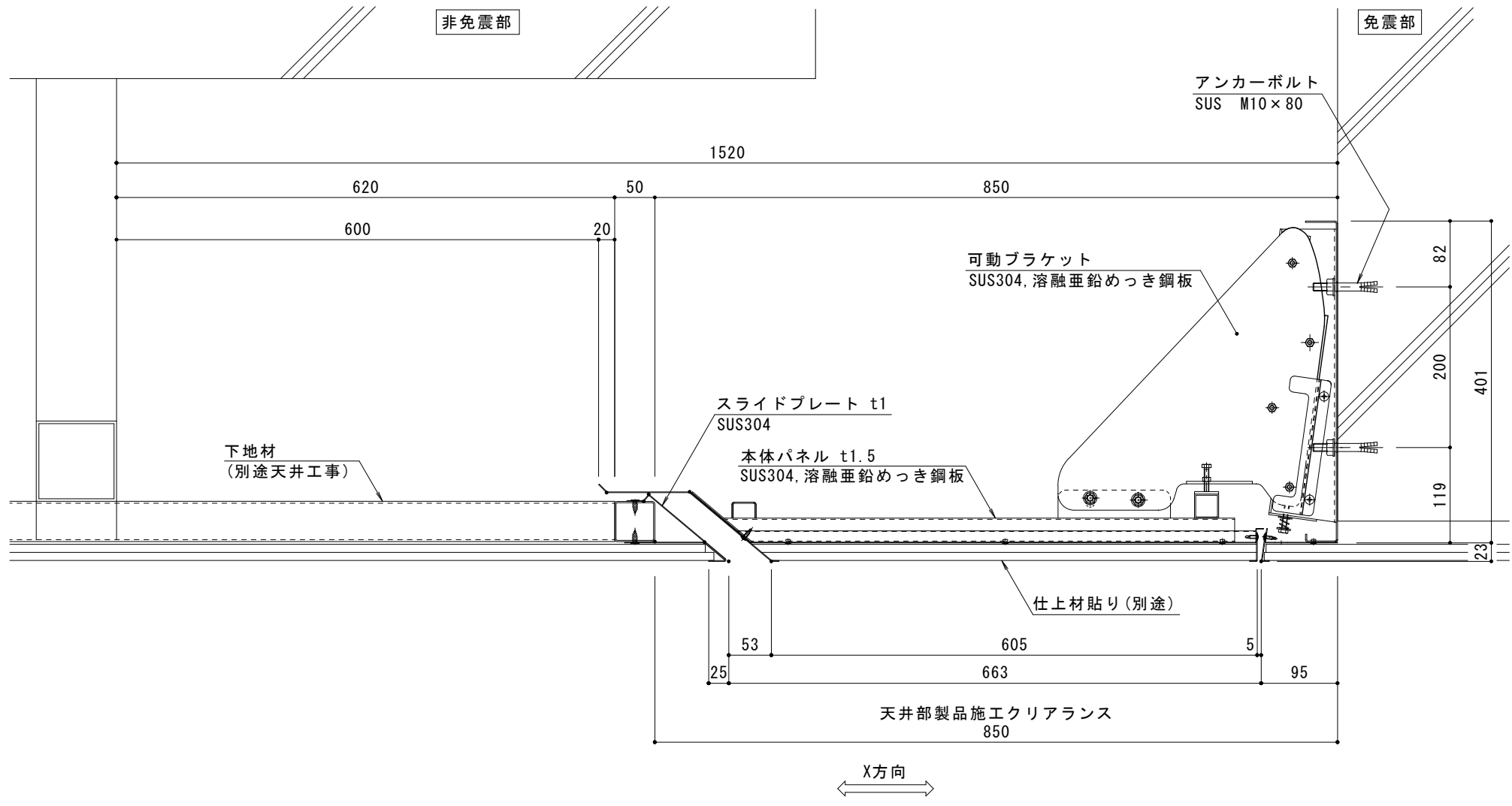
断面詳細図 S = 1 : 5
