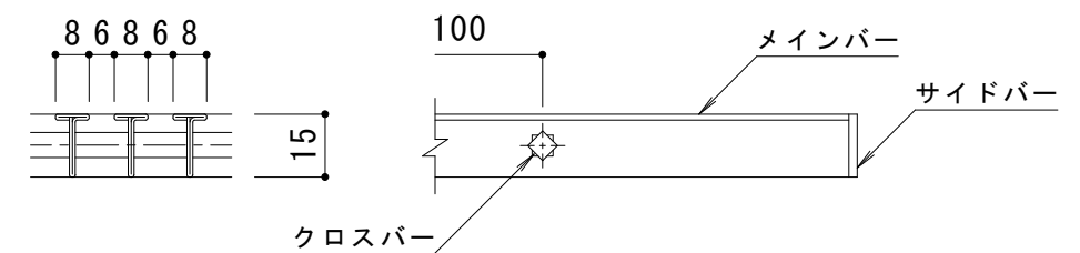
B-B断面図
