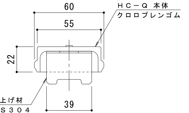
D - D 断面図
