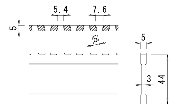
DI-44 バー形状詳細 S=1:2
